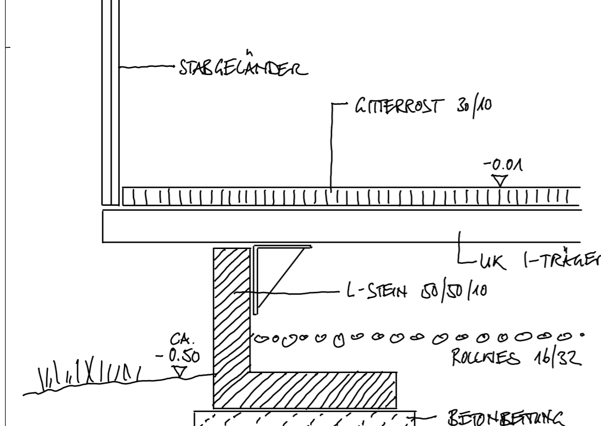
Regelschnitt Aufstellfläche für Müllcontainer Prinzipische Skizze zur Gründung und Konstruktion, die im Detail noch abzustimmen ist. ohne Maßstab
