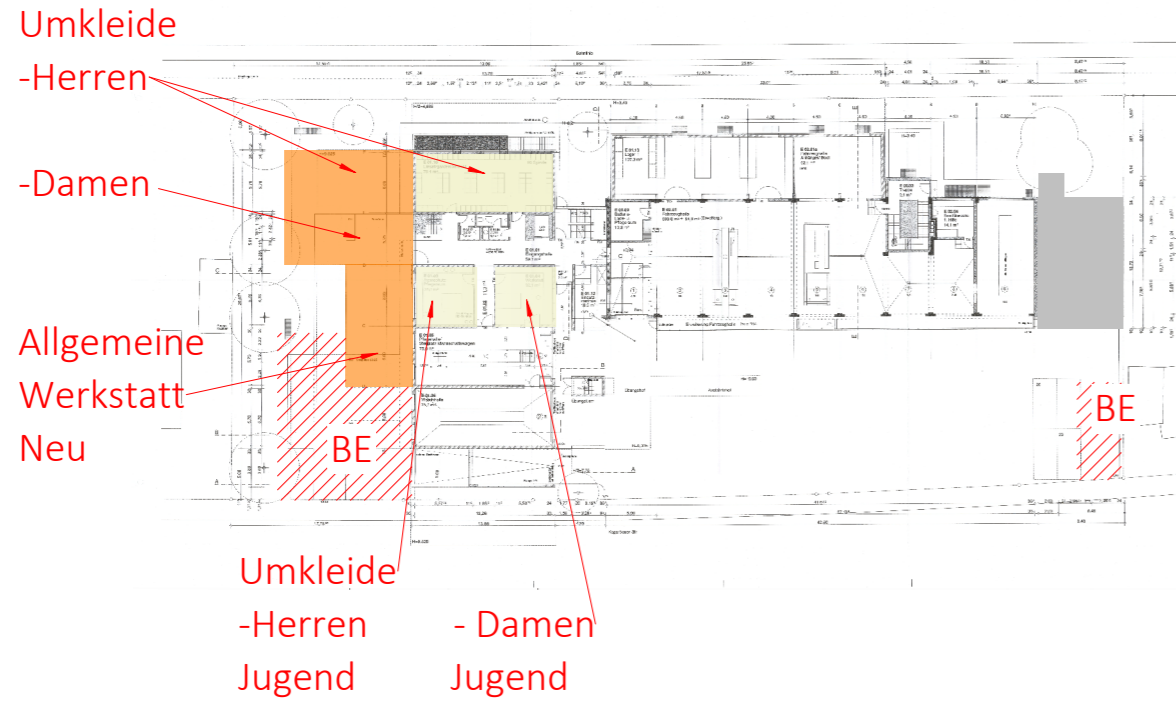
Grundriss EG
